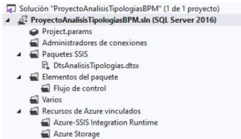
Ilustración 1: Solución AnalisisTipologiasBPM
